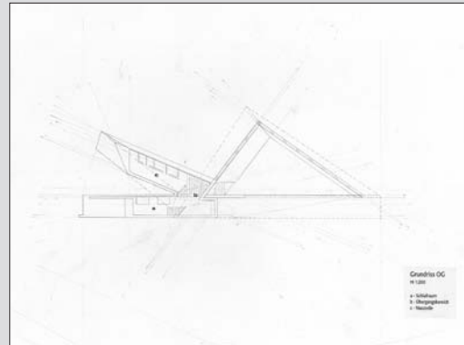
Nutzungsdiagramm und Grundrisse/Schnitt
