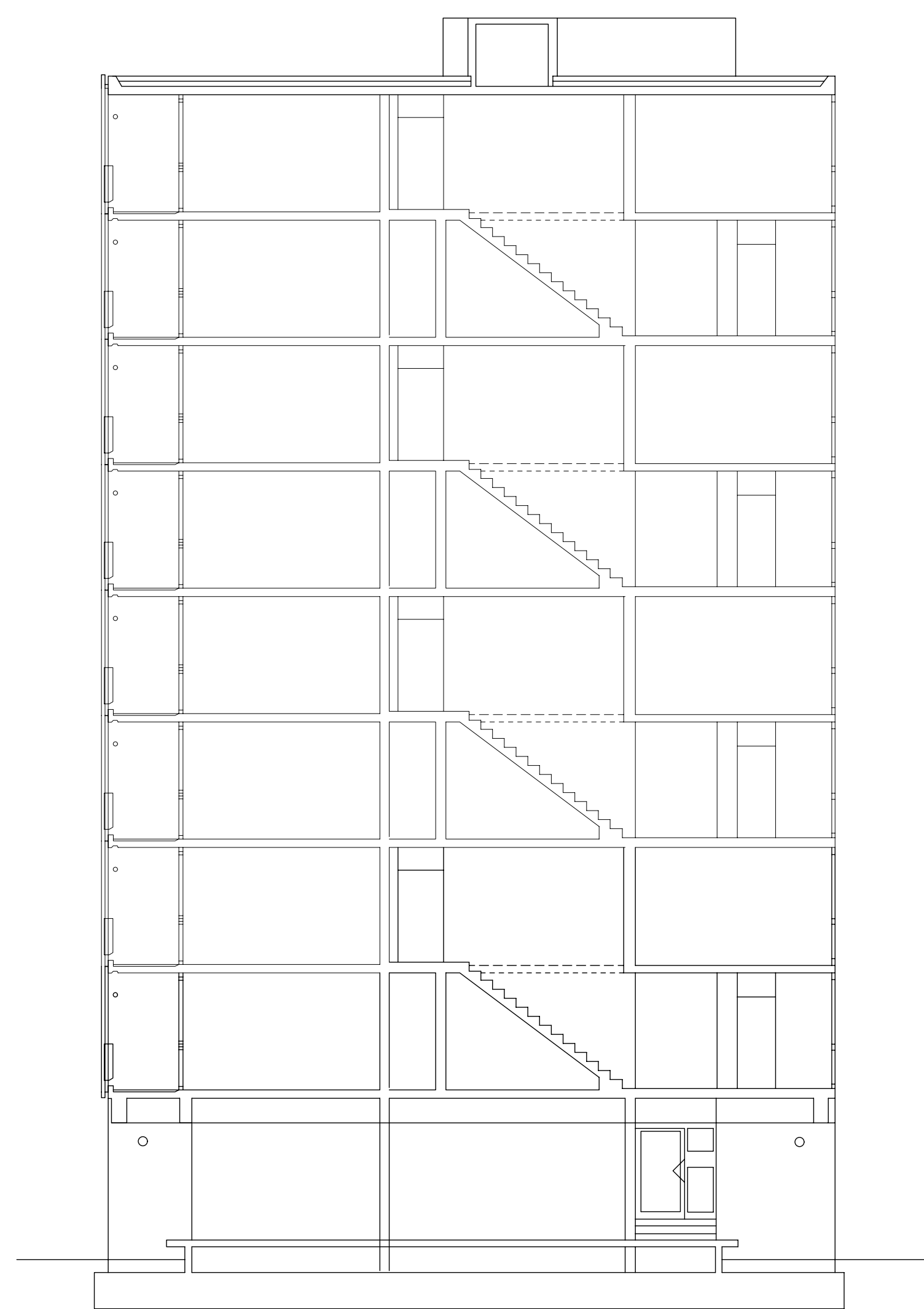
Schnitt 1:100
