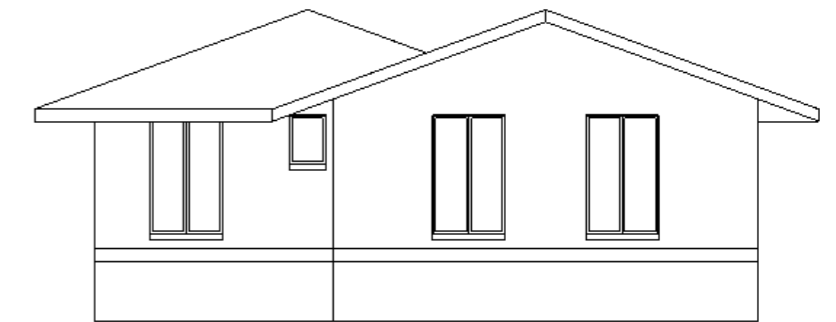
Ostfassade
