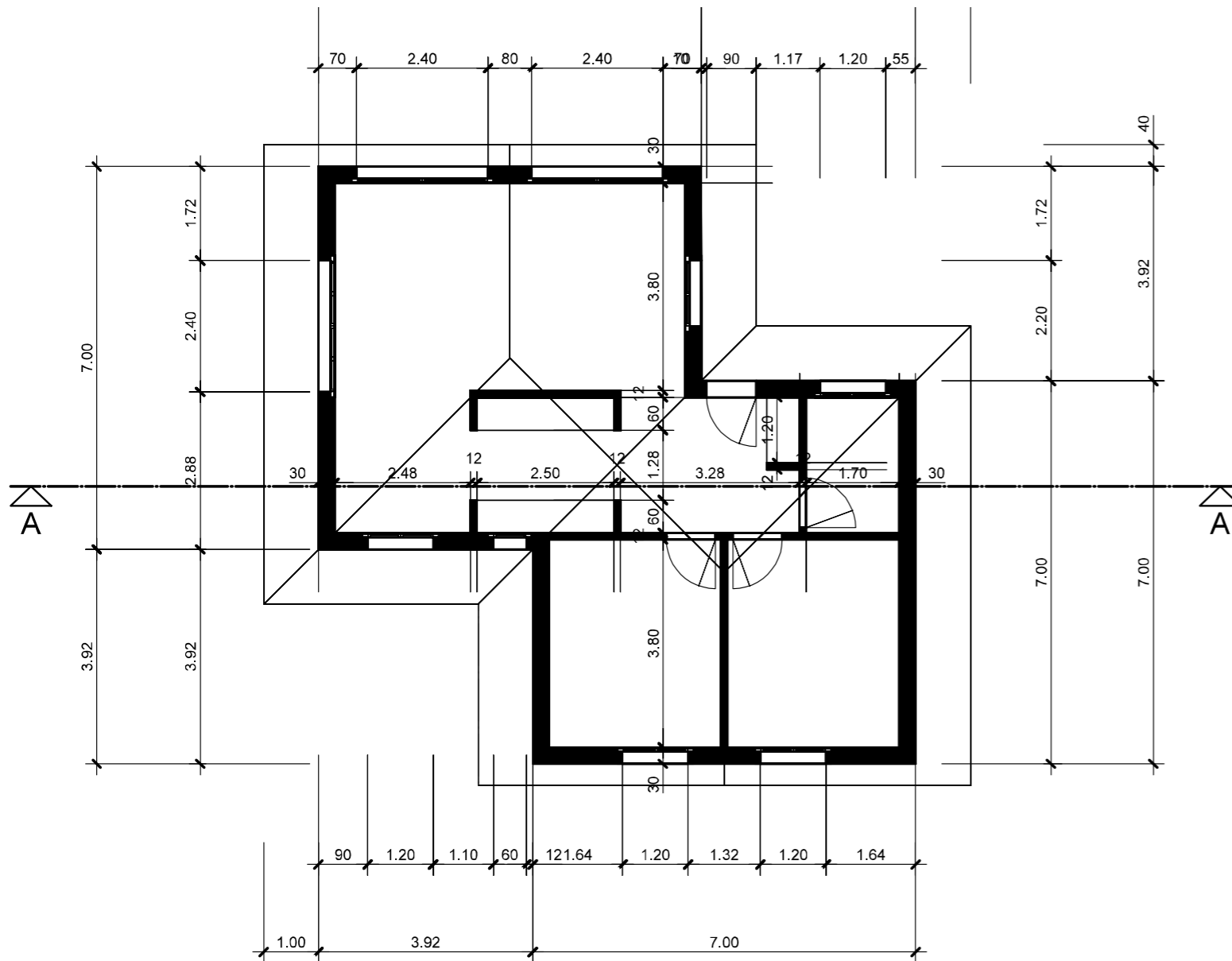
Grundriss
