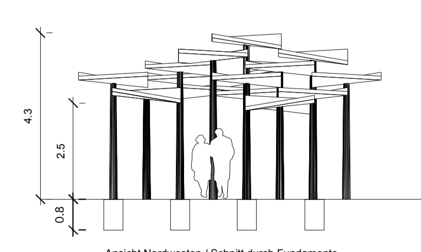
Ansicht Nordwesten / Schnitt durch Fundamente Fundamente: Betonfundament und verankerte Fussplatte
